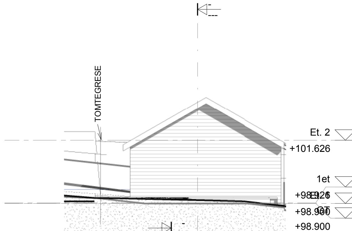
FASADE MOT NORD GARASJEN 1 : 100
