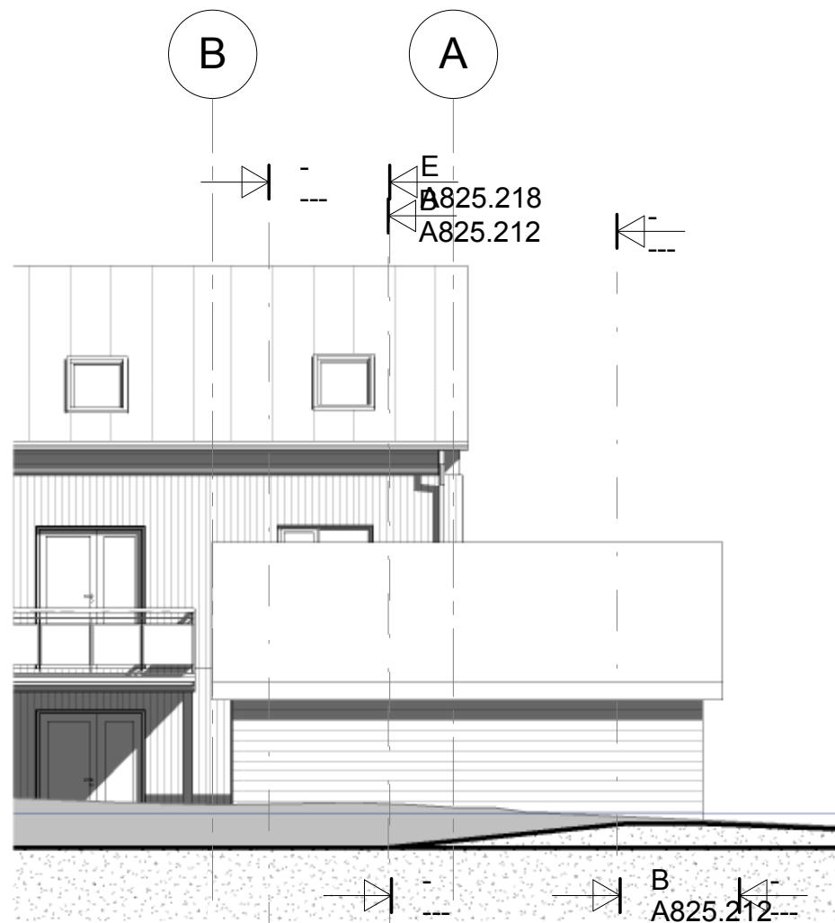
FASADE GARASJEN MOT ØST 1 : 100
