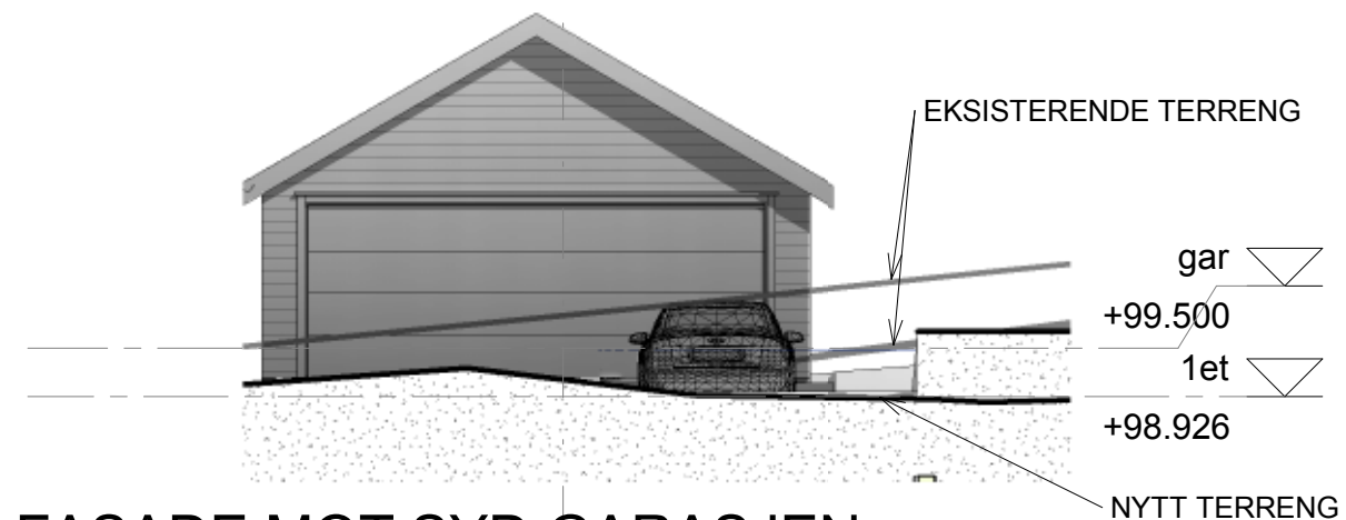
FASADE MOT SYD GARASJEN 1 : 100
