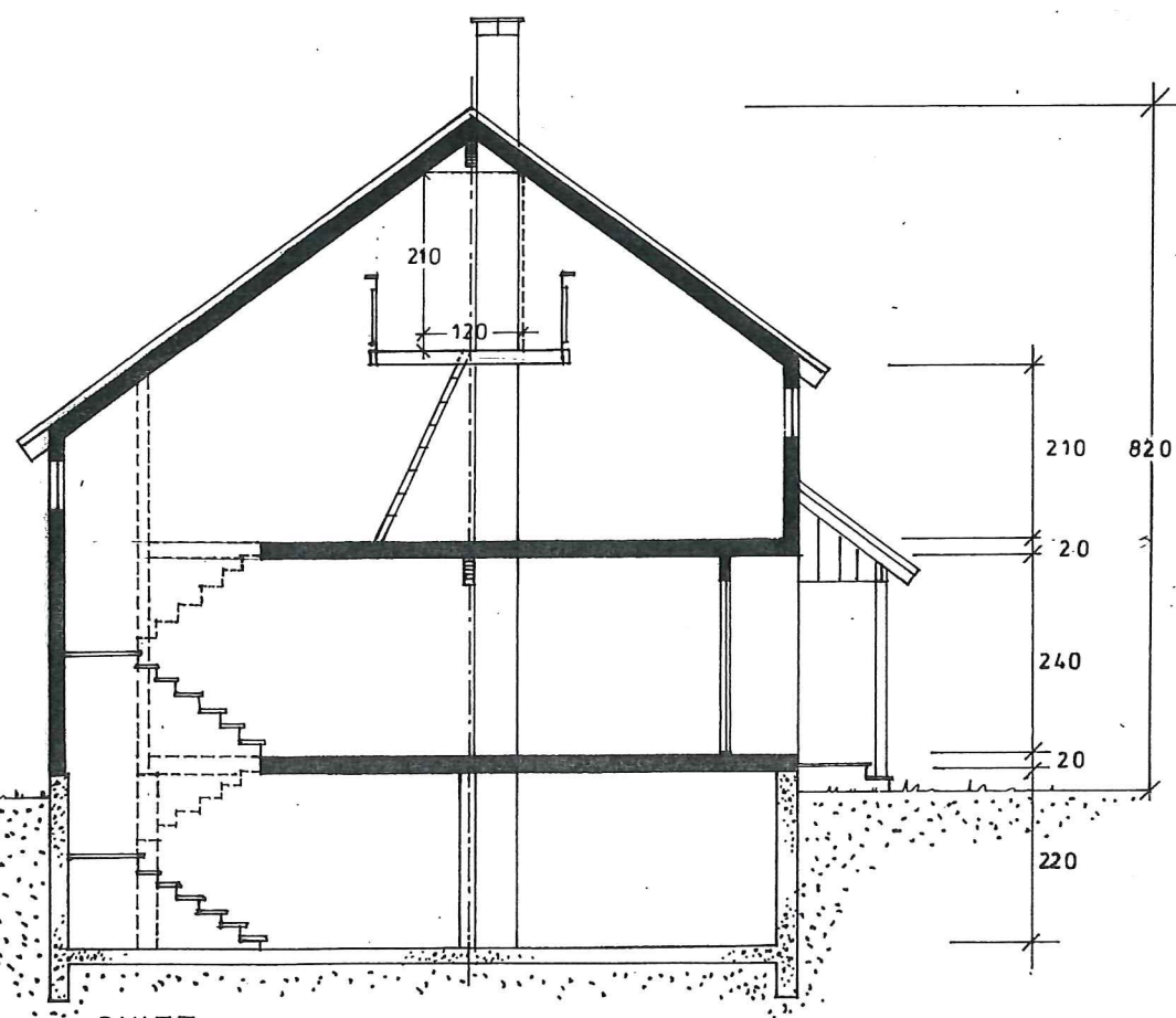
SNITT
